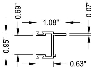
3K VENT JAMB ALUM (6063-T6)
